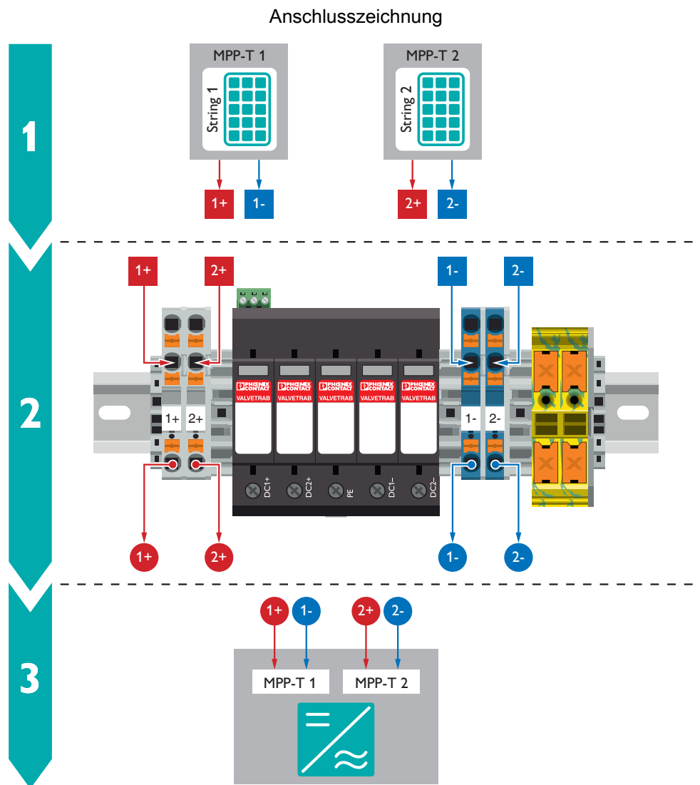
Schematische Applikationszeichnung
