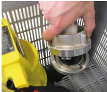
Schlauch anschließen
